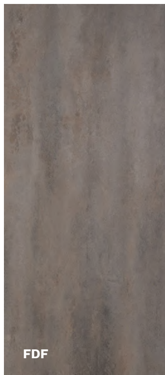
HEMATYT
