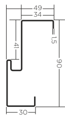
ościeżnica PU56 STANDARD
