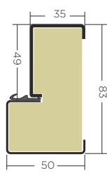
ościeżnica Termo ODS56 ZA DOPLATĄ - 520,00 HIT!
