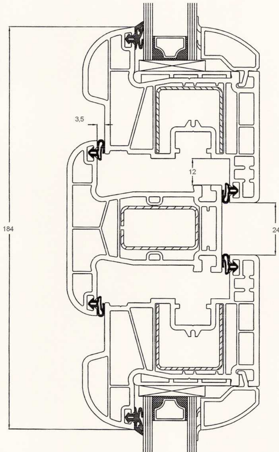
Rys. 15. Przekrój przez ramy skrzydeł i słupki stałe (ślemię) - system AVANTGARDE 9000
