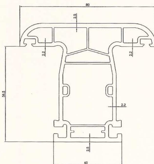
Rys. 3. Kształtownik ramiaka skrzydła 9001 z nieplastifikowanego PVC – system AVANTGARDE 9000
